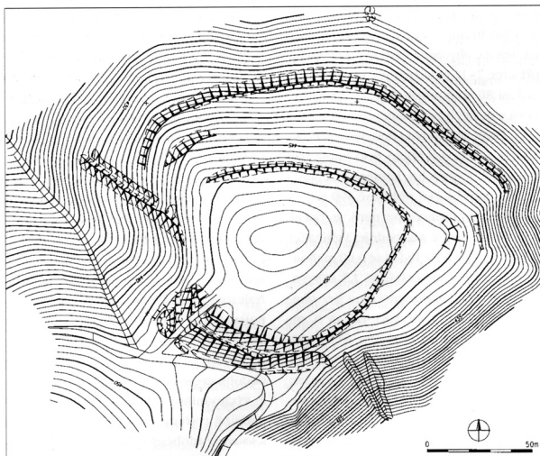
Biskupice. Hradisko nad Nectavou: půdorysný plán lokality (podle DOLEŽEL, Jiří: Biskupice /k. ú. Biskupice u Jevíčka, okr. Svitavy/ . Hradisko nad Nectavou . Přehled výzkumů, 48, 2007).
