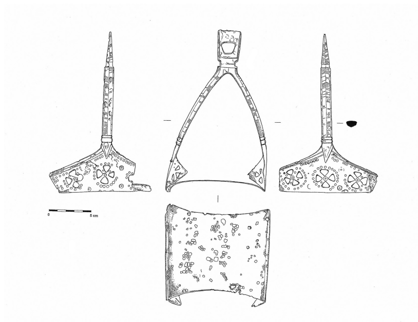
Bělecký mlýn (k. ú. Kladky?, k. ú. Zdětín?): tautovaný prolamovaný železný třmen, inv. č. 142969 (kresba M. Schindlerová).
